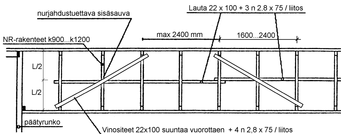
Kuva 14. Yleisohje sisäsauvan nurjahdustuennan toteuttamiselle.
