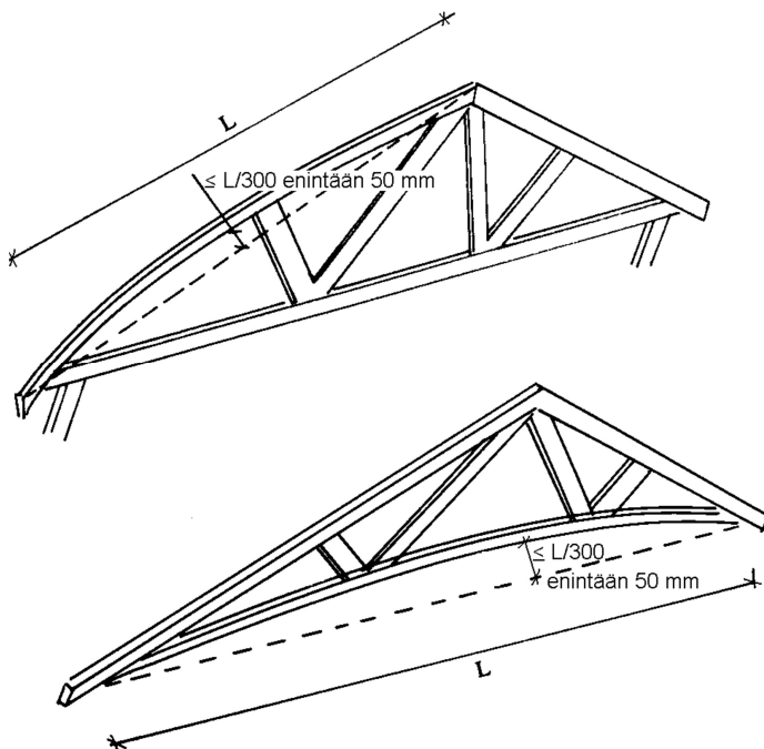
Kuva 6. Paarteiden asennustoleranssit.
