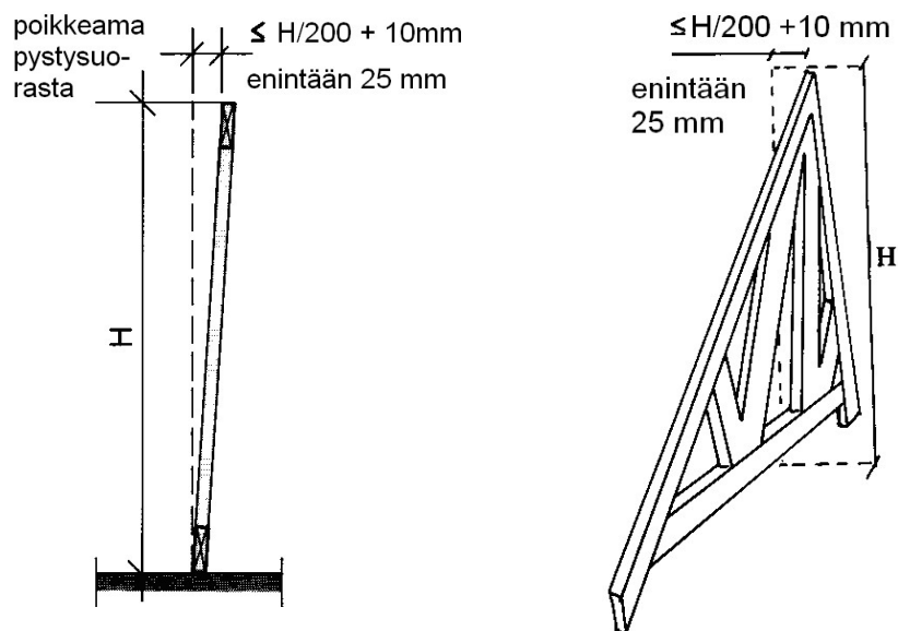
Kuva 7. Pystysuorustoleranssi
