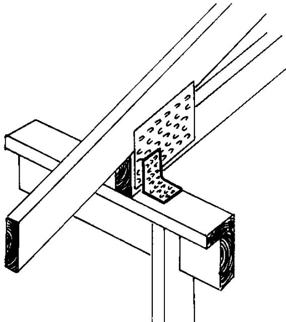
Kuva 12. Tukikiinnitys kulmakiinnikkeellä
